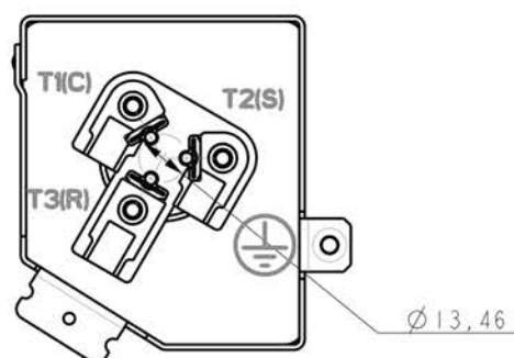
壓縮機接線示意圖
